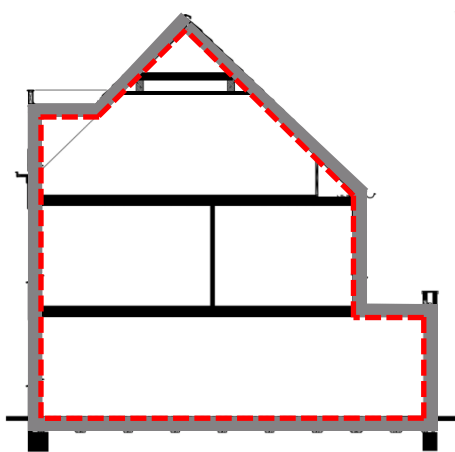
Figuur 2a: Te meten zone valt binnen de thermische schil (= luchtdichte schil); ook de vloering ligt binnen de thermische schil ; vliedluiken behoren tijdens de meting open te zijn; knieschotten behoren tijdens de meting gesloten te zijn – zie hiervoor paragraaf 5.1.5.
