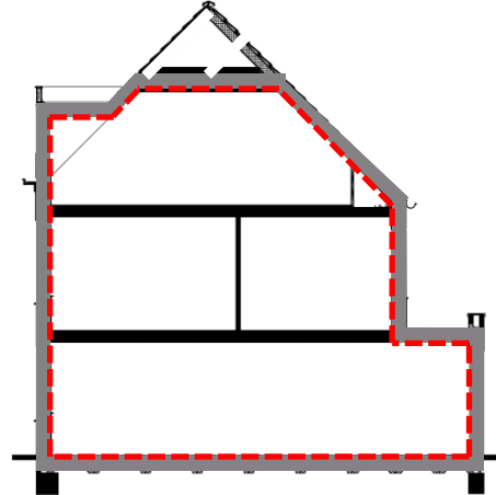
Figuur 2b: Te meten zone valt binnen de thermische schil (= luchtdichte schil); de vloering ligt buiten de thermische schil ; vliedluiken/knieschotten behoren tijdens de meting gesloten te zijn – zie hiervoor paragraaf 5.1.5.
