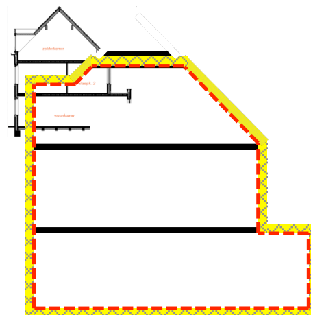
Figuur 2b: Te meten zone valt binnen de thermische schil (= luchtdichte schil); de vloering ligt buiten de thermische schil; vliedluiken/knieschotten behoren tijdens de meting gesloten te zijn – zie hiervoor paragraaf 5.1.5.
