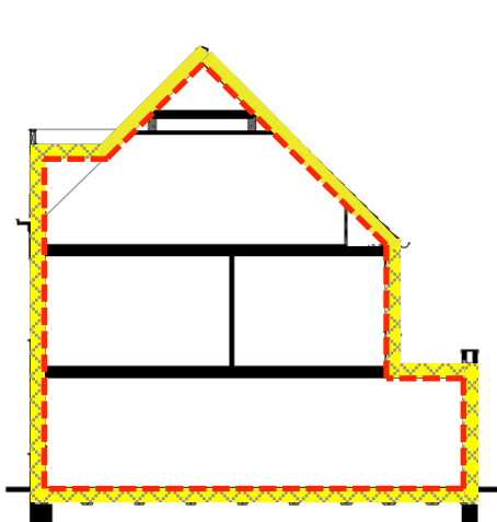
Figuur 2a: Te meten zone valt binnen de thermische schil (= luchtdichte schil); ook de vloering ligt binnen de thermische schil; vliedluiken/knieschotten behoren tijdens de meting gesloten te zijn – zie hiervoor paragraaf 5.1.5.
