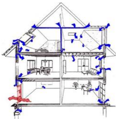
Figuur 2c Gebouwschil: linker figuur luchtlekken/rechter figuur gele arcering is voorbeeld van een luchtdichte schil c.q. te meten zone van het gebouw
